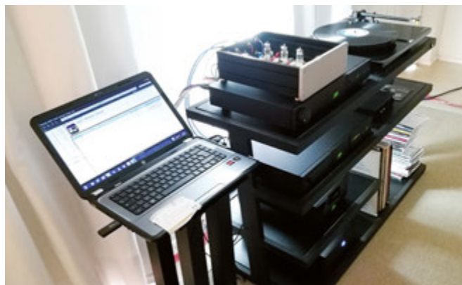
Dimensione Suono di Lucca presentava un ammiratissimo pre-pre autocostruito (dual Jfet e valvole) abbinato a un giradischi Rega P6 con testina Exact, amplificazione Naim NAC152 XS + NAP100 e diffusori Totem Forest. Sorgente digitale Naim CD5XS + DAC V1. Cavi Rega, QED e Nordost Red Down LS.
